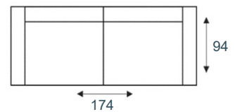
2,5-zitsbank 2 pl/02
