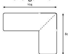
bovenaanzicht
