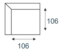
hoekelement CORNER
