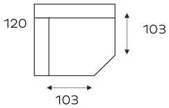
HOEKELEMENT LI | RE HOEK LI/RE 120
